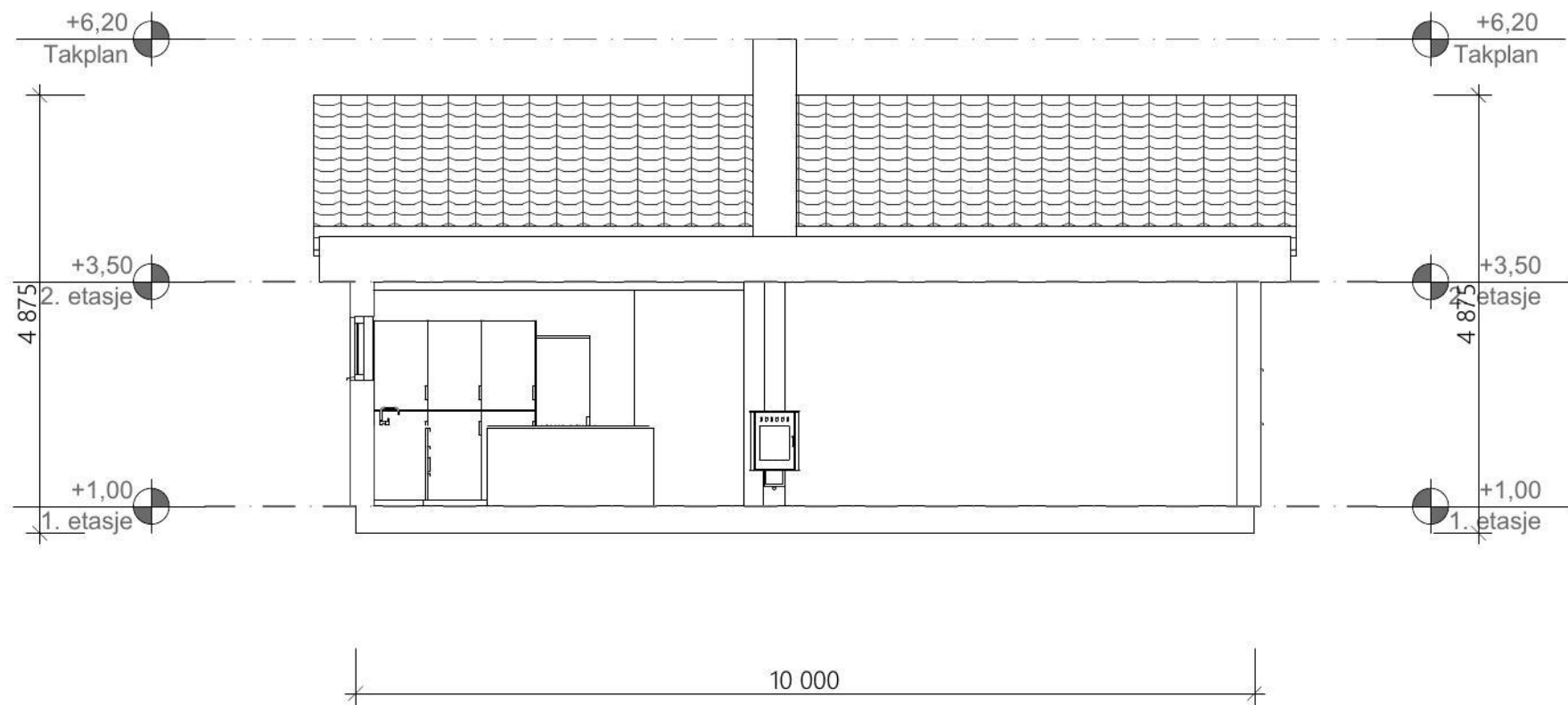
1:100 Snitt A
