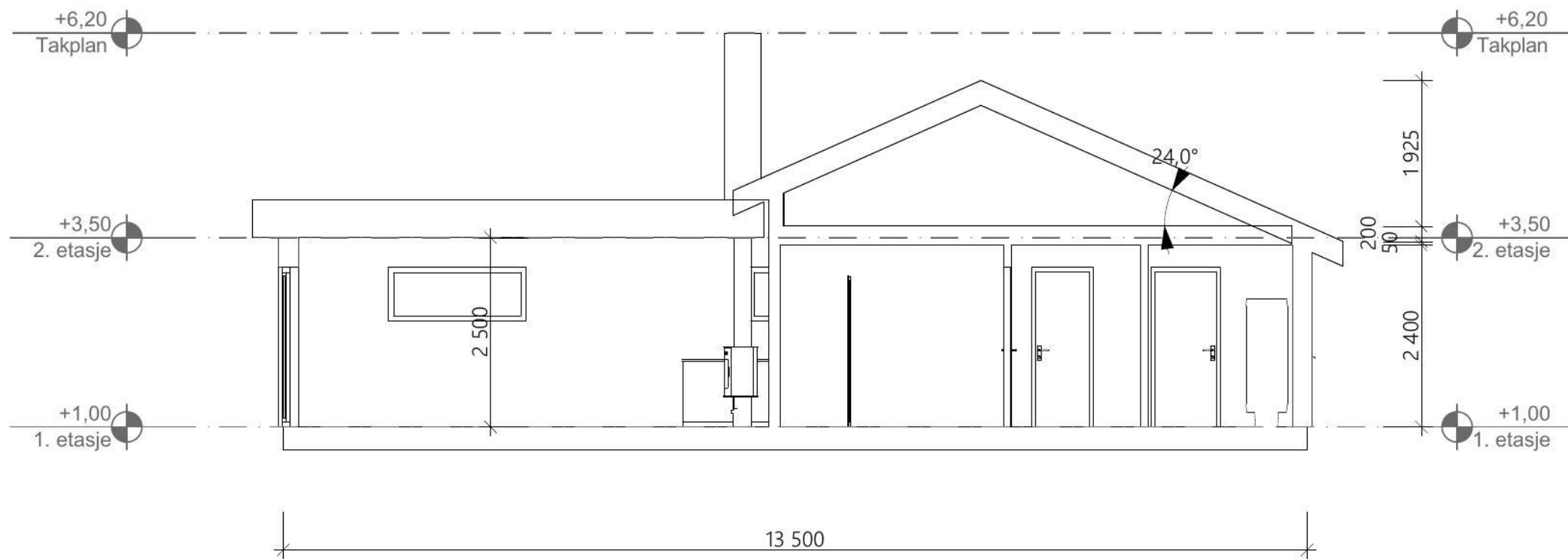
1:100 Snitt B
